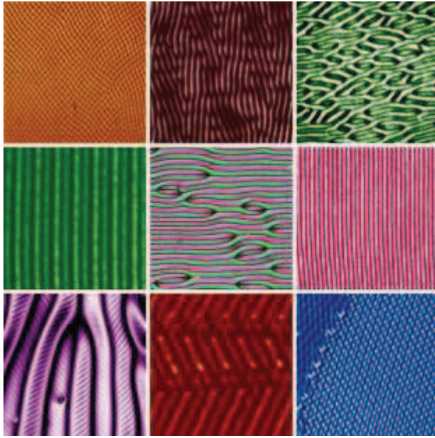
2. ábra. Elektrokonvekciós mintázatok folyadékkristályban
